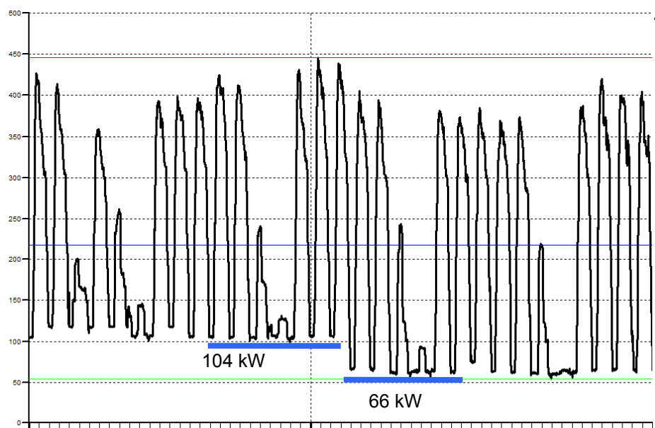
Monats-Lastprofil Stromzähler Bildungs- und Verwaltungszentrum (Oktober 2013)
